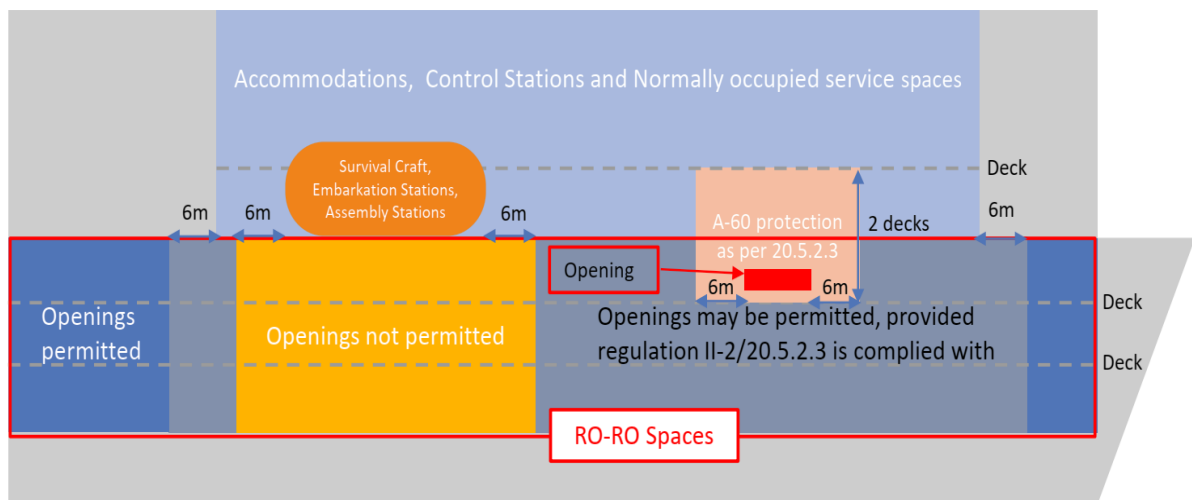
로로 여객선 상 허용가능한 개구의 배치
